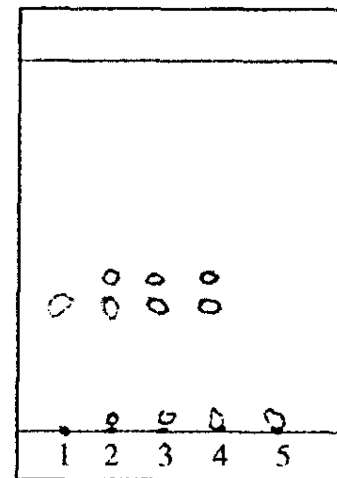
1. 补骨脂素对照品;2-4. 样品;5. 空白(空补骨脂)
