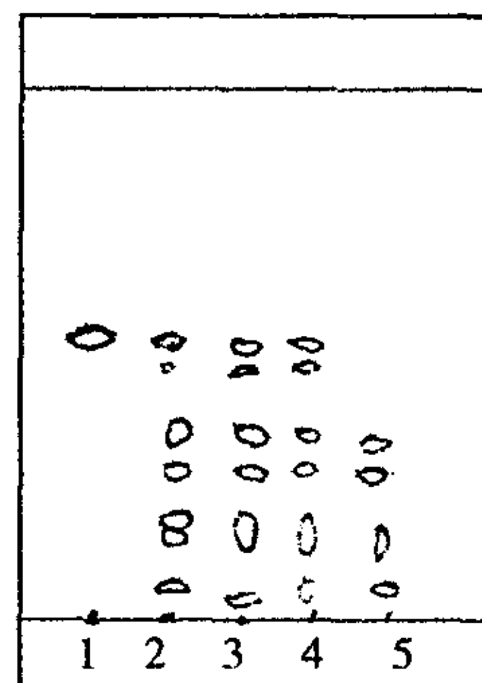
1. 原儿茶醛对照品;2-4. 样品;5. 空白(空丹参)
